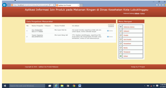
Gambar 16 Halaman Pengaduan
