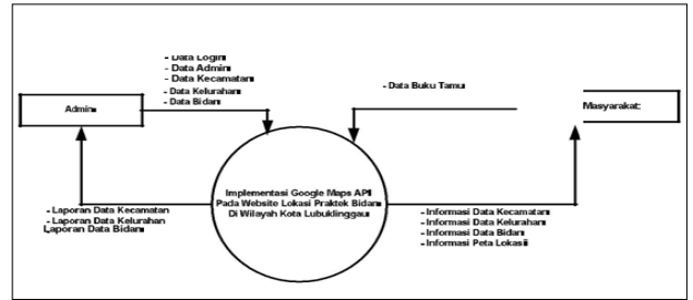
Gambar 2. Diagram Konteks
